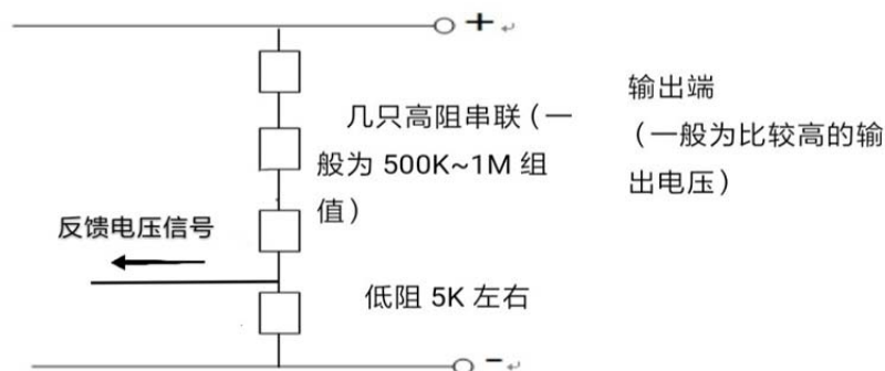
图 16 串联分压反馈电路
