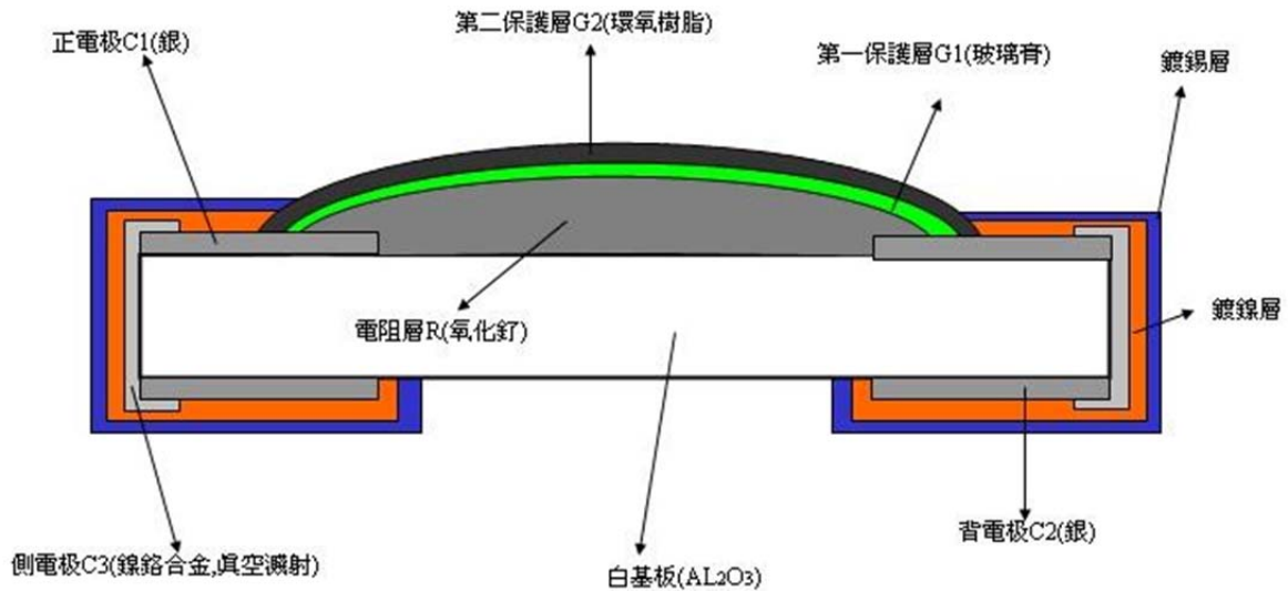
图 6 电阻使用前结构图
