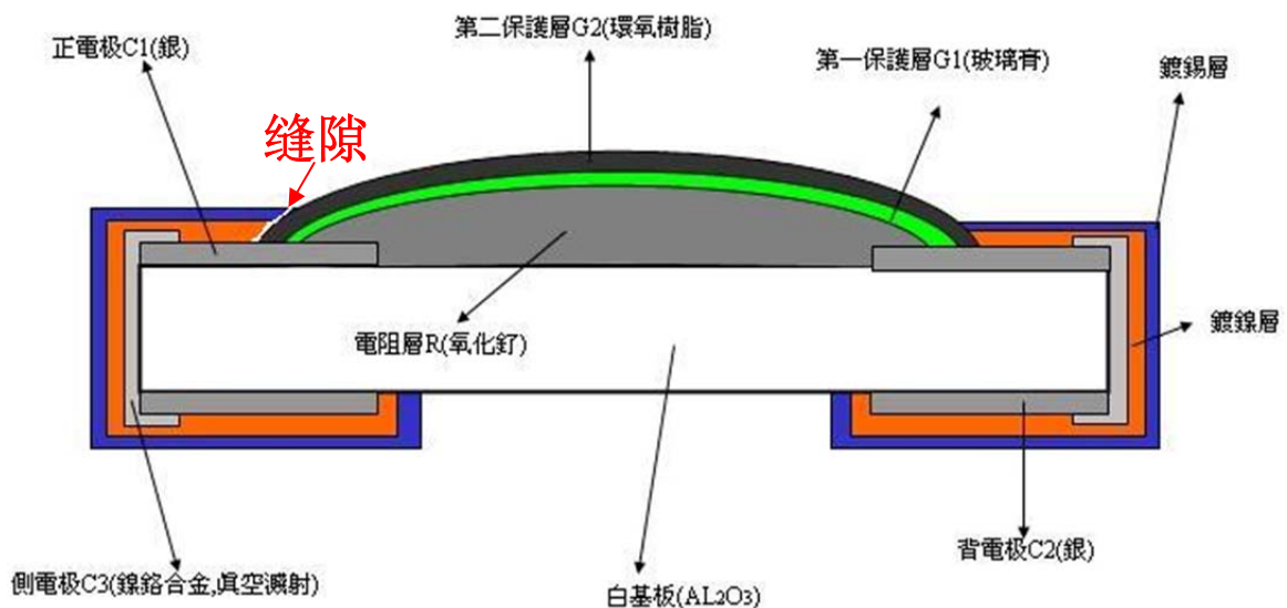
图 7 使用后电阻结构图
