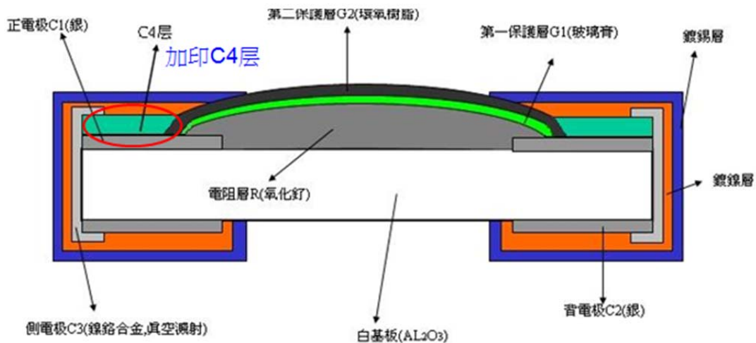
图 17 抗硫化电阻器结构图
