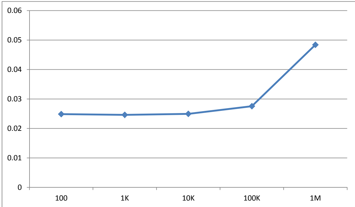
图表 4: MS12 10mΩ 不同频率电流下阻值测量平均值折线图
