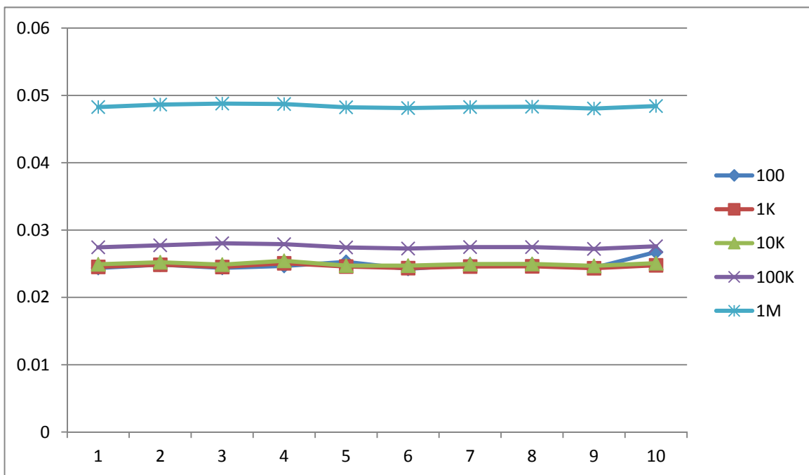
图表 3: MS12 10mΩ 不同频率电流下阻值测量折线图
