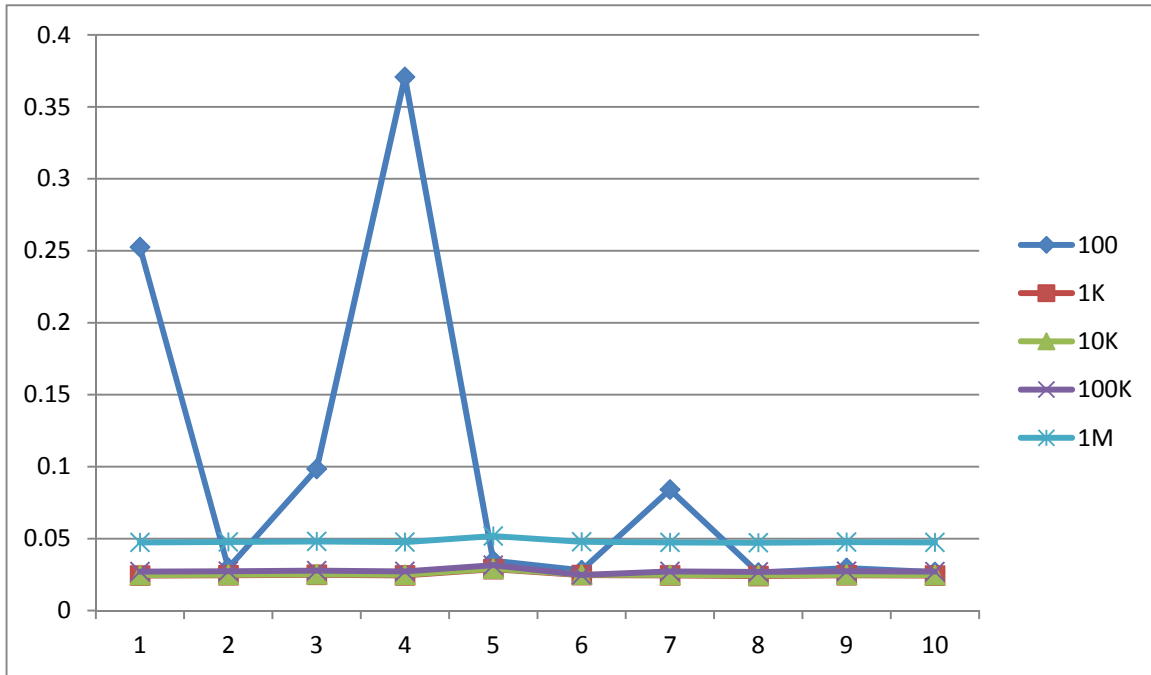
图表 1: MS06 10mΩ 不同频率电流下阻值测量折线图
