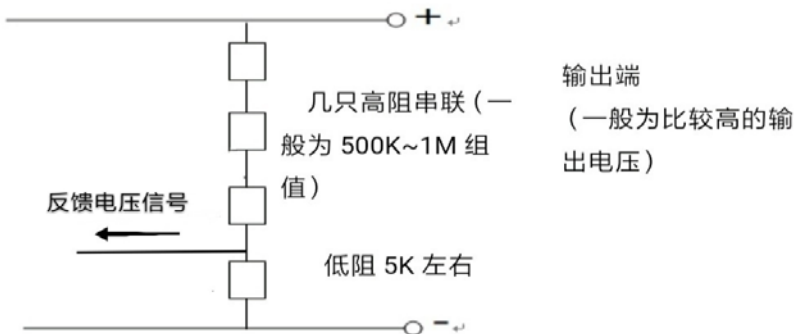
图 15 串联分压反馈电路
