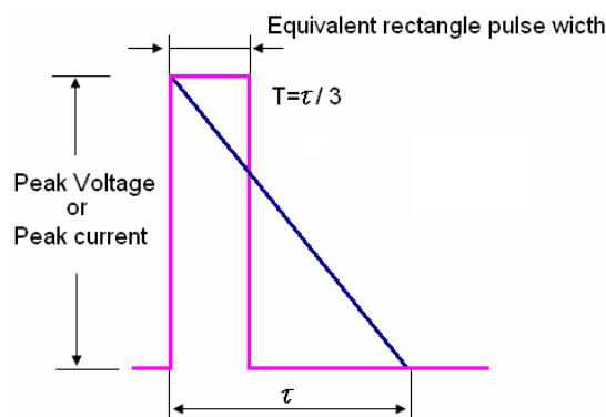
b. 三角波形
