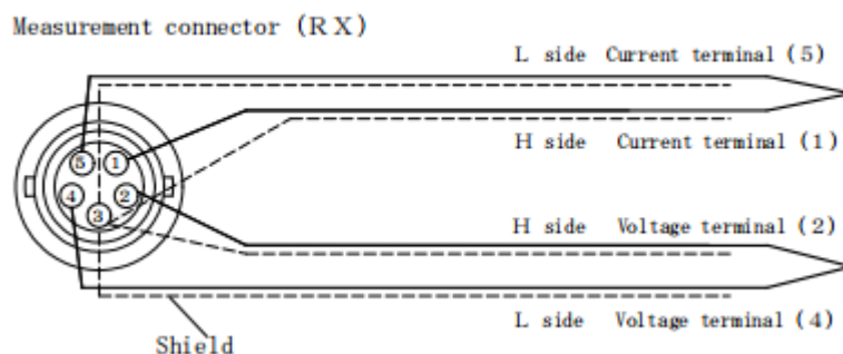
测量仪表连线
