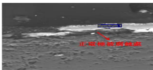
图 3 正电极交接处
